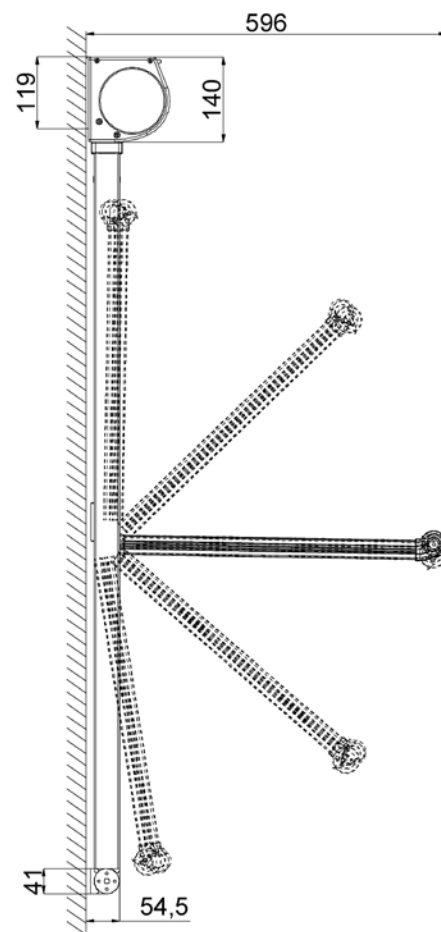
Installazione a parete con braccetti
