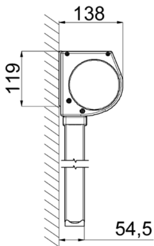
Installazione a parete
