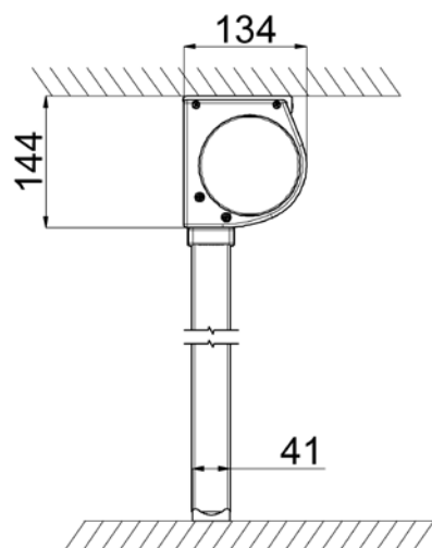
Installazione a soffitto
