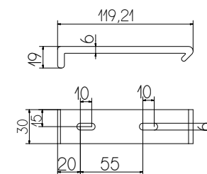
Staffe cassonetto
