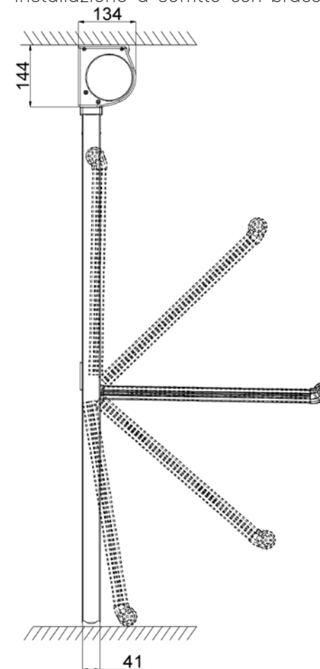
Installazione a soffitto con braccetti
